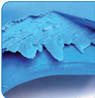
Quand le PVC de structure amorphe (section inférieure) est soumis au processus d'orientation, on a comme résultat une structure laminaire (section supérieure).
