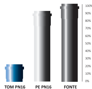
Coût de l'installation (euro/m)
