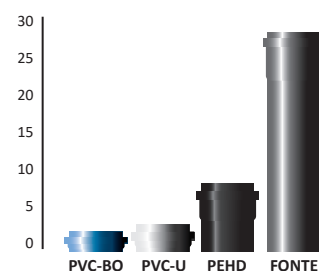
Énergie consommée en pompage en 50 ans (kWh)
